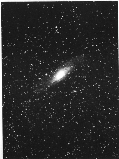
Galassia di Andromeda con le due piccole galassie compagne M31 ed M32. La ripresa è stata effettuata in località Alpe Giumello in provincia di Como il 21 ottobre 1976, tempo di esposizione di nove minuti con pellicola Kodak 103 aF. (Foto di Luigi Piatti e Lorenzo La Rocca).
